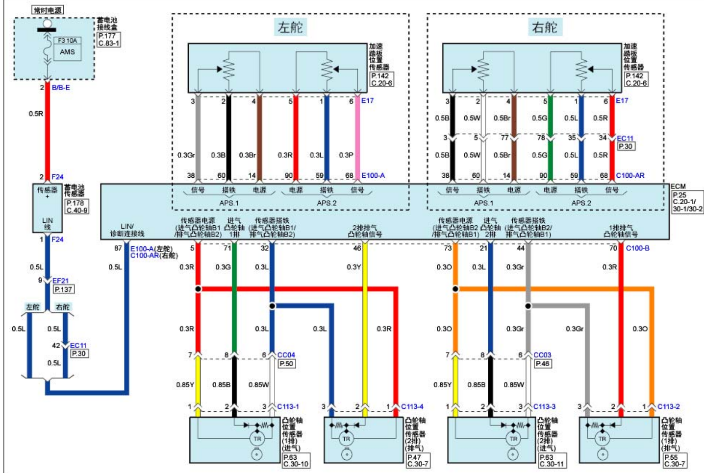
发动机控制系统(G6DG/G6DH/G6DJ:LAMBDA II 3.0L/3.3L/3.8L GDI)(10)
